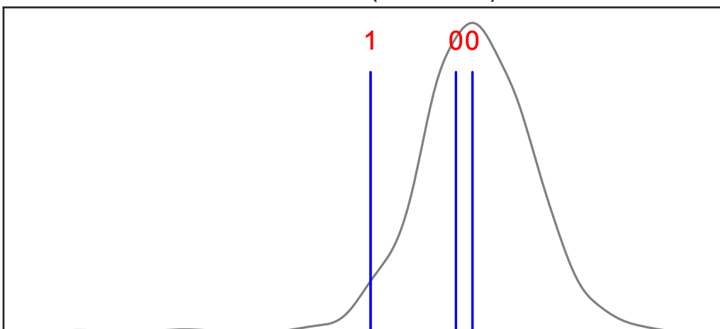
TRIM67 (Katsano)
