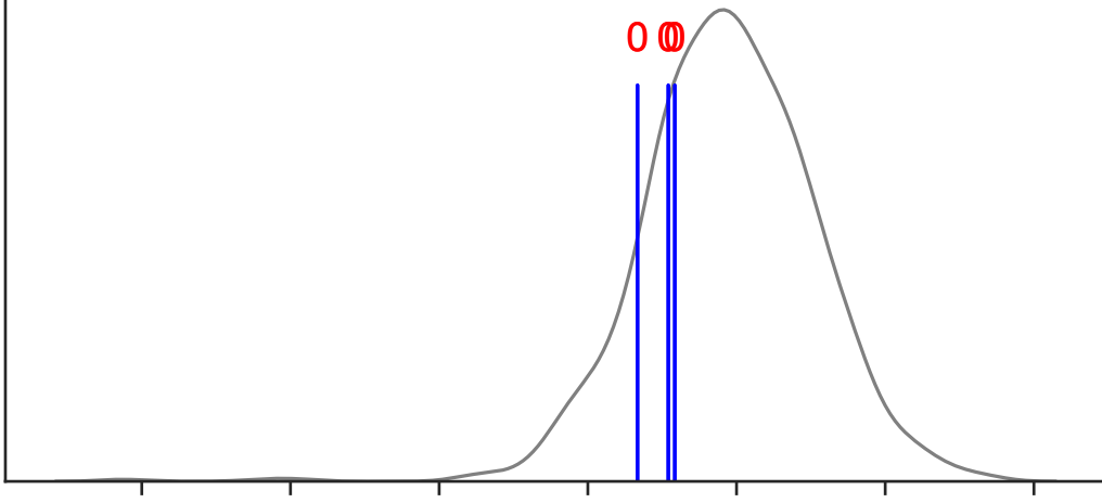
COL20A1 (Katsano)
